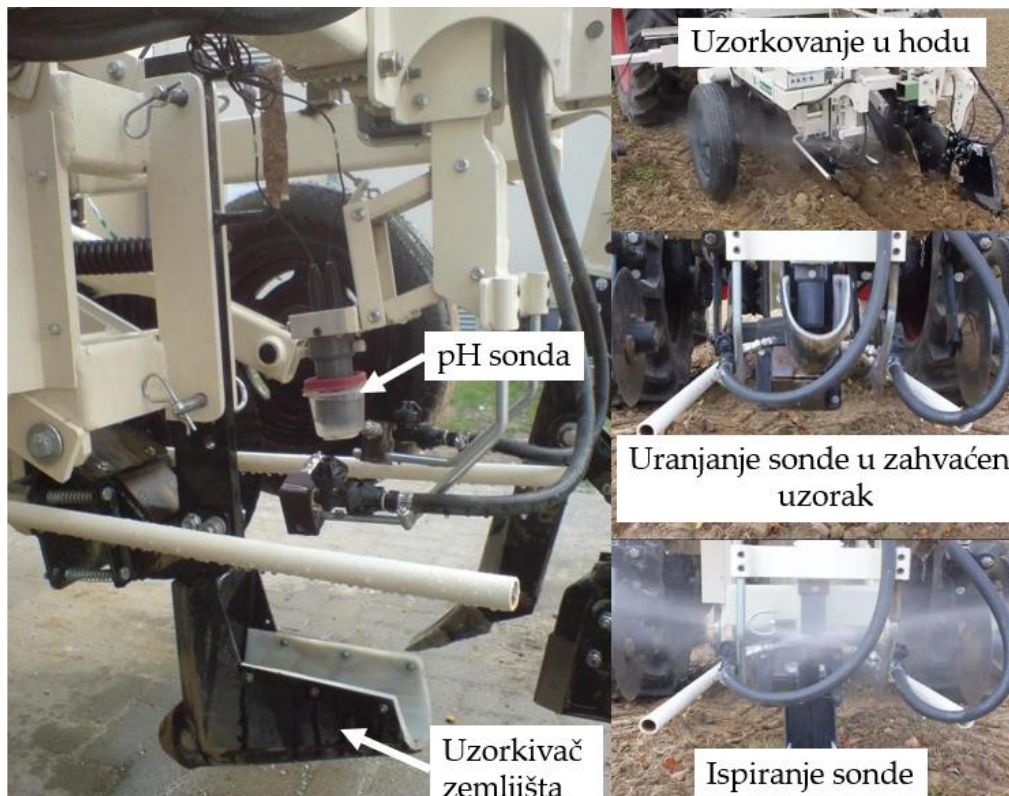
Slika 1.18. Senzorski sistem (ISFET) za mapiranje pH, električne provodljivosti i spektralne karakteristike
